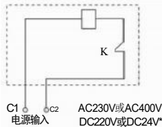
图4：分励脱扣器接线图
