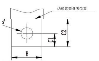
图2铜排及开孔尺寸示意图
